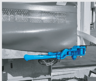
Tension arrière de rideau par cliquet
